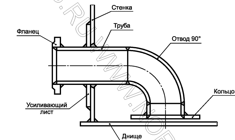
а) Патрубок со сварным присоединением отвода
