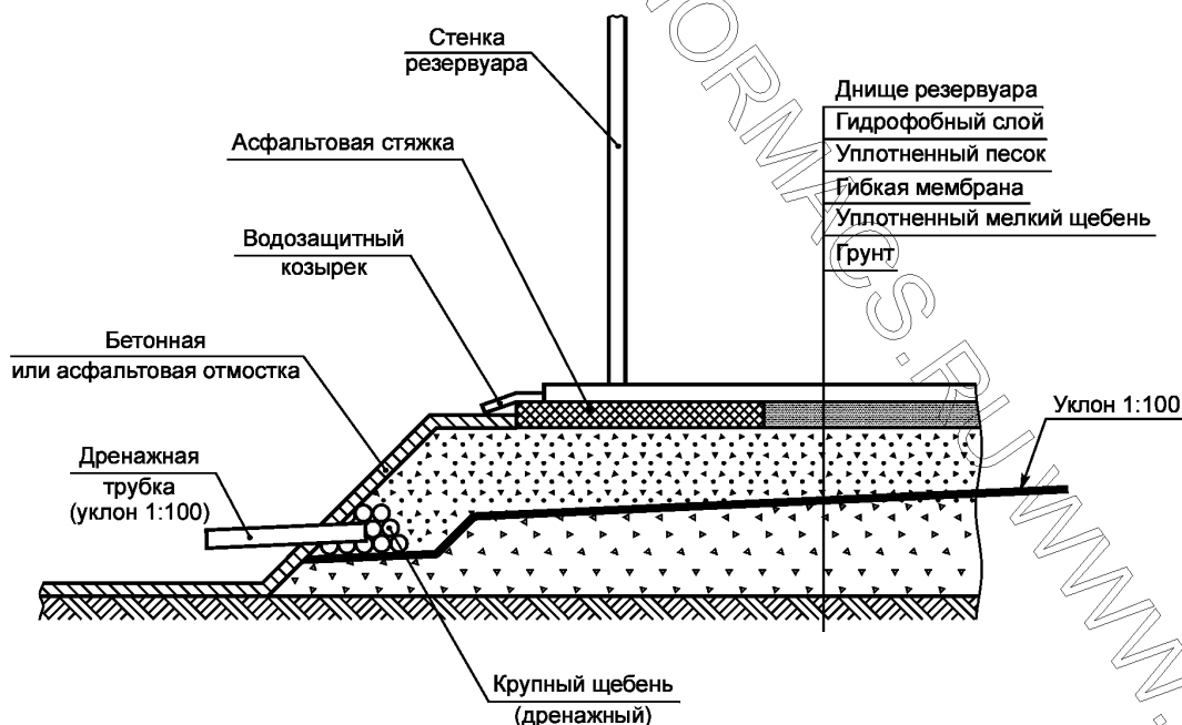
Рисунок 24 — Грунтовая подушка
