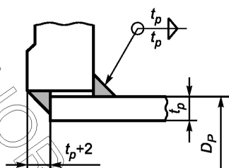
Рисунок 12 — Соединение фланца патрубка с обечайкой (трубой)
