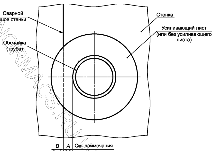
Пересечение шва стенки усиливающим листом
