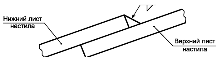
Рисунок 7 — Нахлесточное соединение листов настила крыши в направлении по уклону крыши
